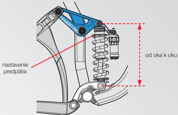
obrázok 1 - pružinový tlmič (Faith)
