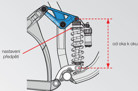
obrázek 1 - pružinový tlumič (Faith)
